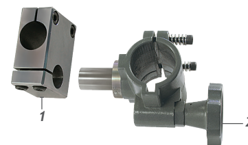
01 - 0801.1115 - Suporte para Tocha MIG/MAG e Plasma 02 - 1400.5013 - Suporte da Cremalheira ø35mm
