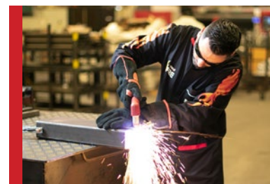
Controle avançado de arco piloto aumentando a vida útil dos consumíveis
