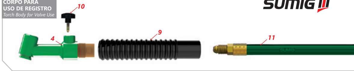
CORPO PARA USO DE ACIONAMENTO Torch Body for Trigger Use
